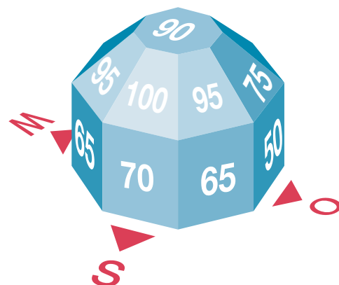
Relativer Stromertrag bei unterschiedlicher Ausrichtung
